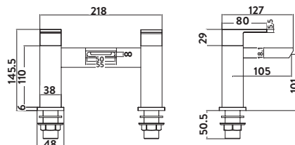
Bath Filler
